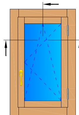
VISTA INTERNA
